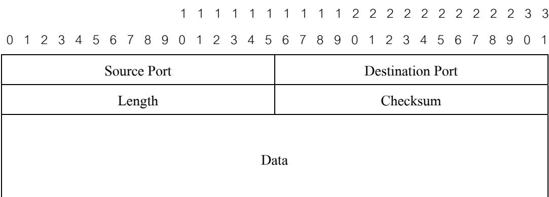
รูปที่ 3-5 แสดงแพ็กเก็ตยูดีพี
